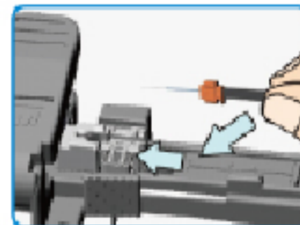
光纤插入连接器
